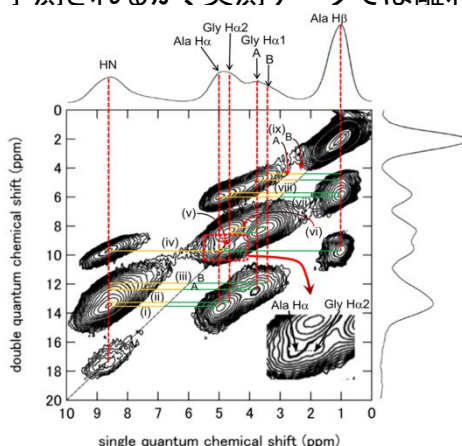
Fig.2 Silk II構造を有する(AG) 15 の固体 1 H DQ-MAS NMRスペクトル
