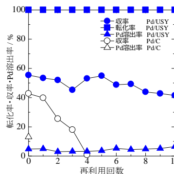
Figure 2 . Pd/CおよびPd/USY触媒における繰り返し反応結果.
